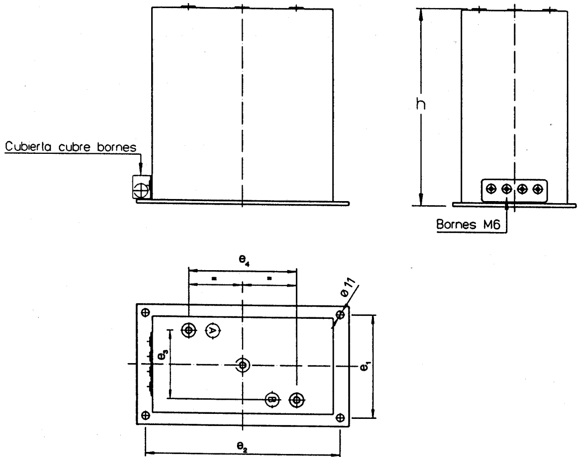
Figura 1. Dimensiones en mm de los transformadores de interior
