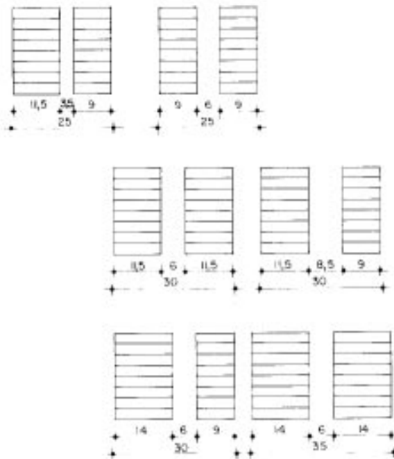
Figura 4.19 - Muros capuchinos cotas en cm
