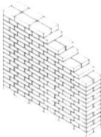
Figura 4.1 - Muro aparejado
